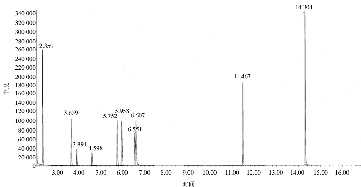
图 F.1 有机挥发物 GC/MS 总离子流图
