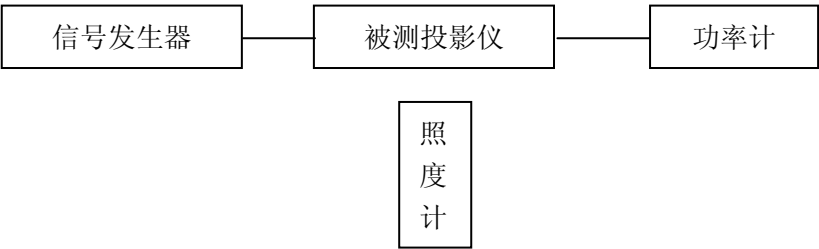
图 A. 3: 工作模式下能耗测试框图
